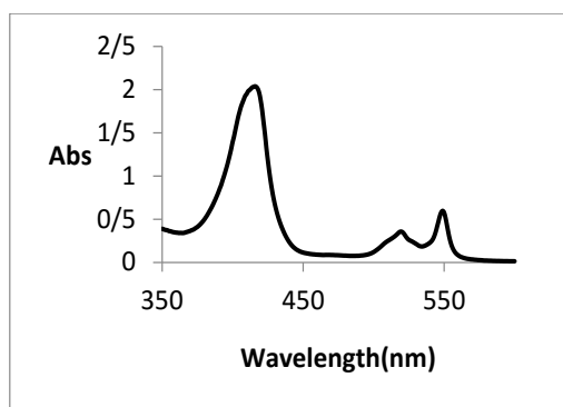
نمودار (۱) UV - طیف مربوط به ۳ پیک جذب سیتوکروم C در حالت احیاء
