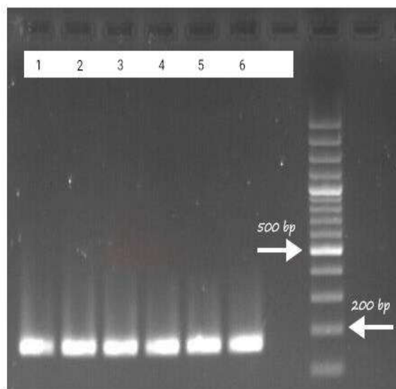
شکل ۵. ژل الکتروفورز آگارز ۱/۵ درصد توالی بورخولدريا در ساین قطعه ۱۹۷ جفت باز 1)NTC 2)10ng 3)1ng 4)100pg 5)10pg 6)1pg همان طور که مشاهده می شود تک باند در ناحیه ۲۰۰ جفت بازی قابل مشاهده هستند. ساین قطعه ۱۹۷ جفت باز است.
