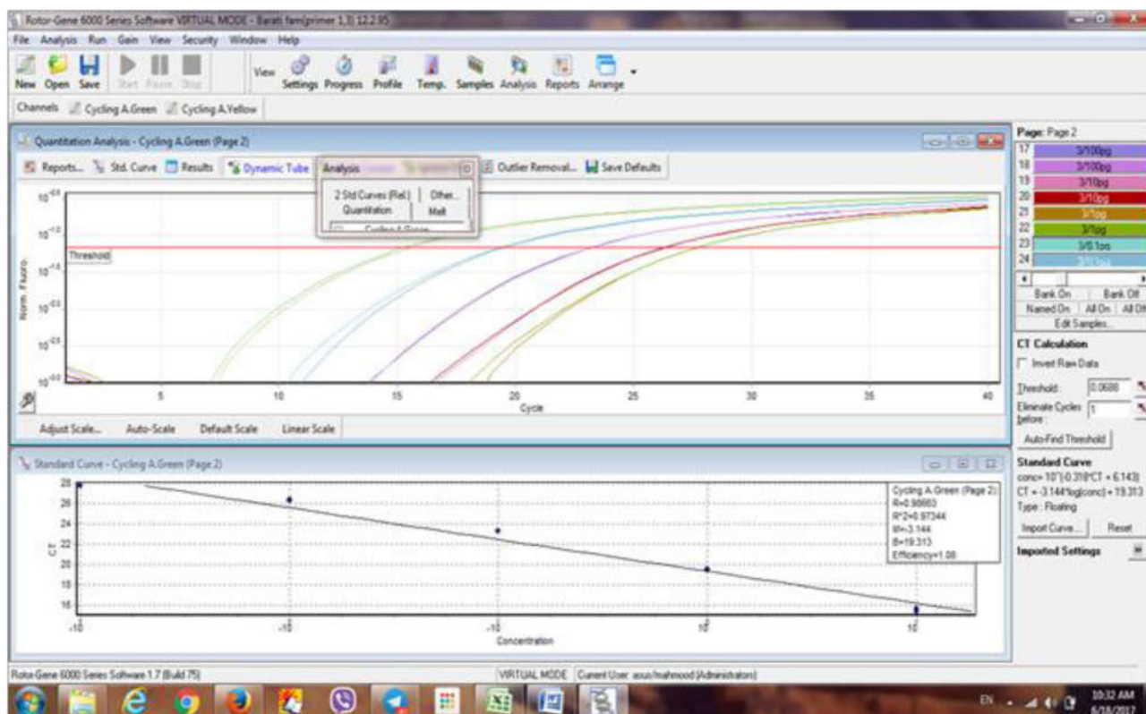
شکل ۴- نتیجه Real-Time PCR با دستگاه Corbett Rotorgene 6000 با استفاده از روش TaqMan مربوط به واکنش پرایمر پیشرو و پیرو و پروب توالی بورخولدريا در غلظت و رقت های مختلف ۱۰۰ نانوگرم، ۱۰ پیکوگرم و ۱ پیکو گرم پلاسمید ۱ همراه نمودار standard curve نکته: هر واکنش به صورت دوگانه انجام شده است و همچنین دارای نمونه کنترل منفی نیز است
