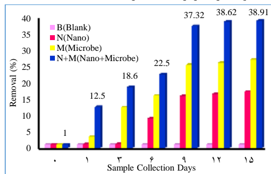
شکل ۷- میزان حذف C 16 در روش آنالیز تبخیری توسط نانوذرات میکروب و g-C 3 N 4
