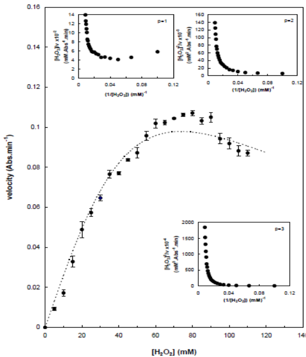
شکل ۵- منحنی اشباع سینتیکی آنزیم پراکسیداز در حضور غلظت های مختلف سوبسترای پراکسید هیدروژن در دوره خواب. نمودار های کوچک بر اساس معادلات سینتیکی پیشرفته برای تعیین تعداد جایگاه های اتصال سوبسترا بر روی آنزیم رسم شده است.
