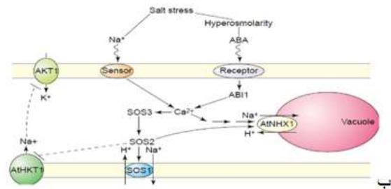
شکل ۱- موقعیت ژن sos1 بر روی کروموزوم شماره ۲ گیاه آرابیدوپسیس (الف)، مسیرهای پیام‌رسانی تنظیم کننده بیان و فعالیت‌های ناقلین یونی جهت حفظ غلظت ناچیز Na^+ در سیتوپلاسم تحت شرایط شوری (ب)
