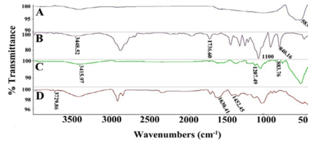
شکل ۳. طیف FT-IR (A) نانو ذرات Fe_3O_4 ، (B) COOH-PEG ، (C) نانو ذرات Fe_3O_4 / COOH-PEG ، (D) COOH-PEG نانو ذرات Fe_3O_4 لود شده با سیس پلاتین می باشد.
