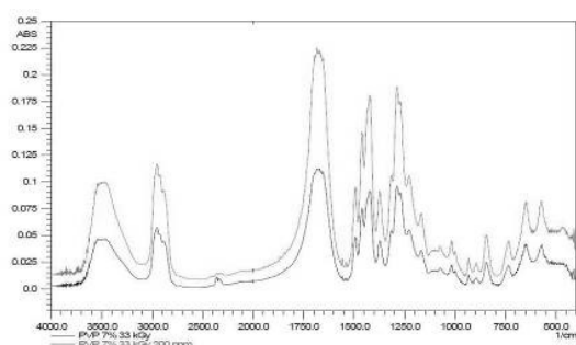
شکل ۴- طیف FTIR در محدوده ۴۰۰۰-۴۰۰ /cm ۱ هیدروژل Ag/PVP با غلظت نقره ۲۰۰ ppm (A) و هیدروژل خالص (B).
