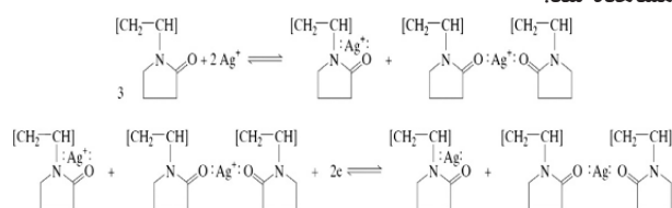
شکل ۵: پیوند کئوردینانس امکان پذیر بین PVP و AgNPs.
