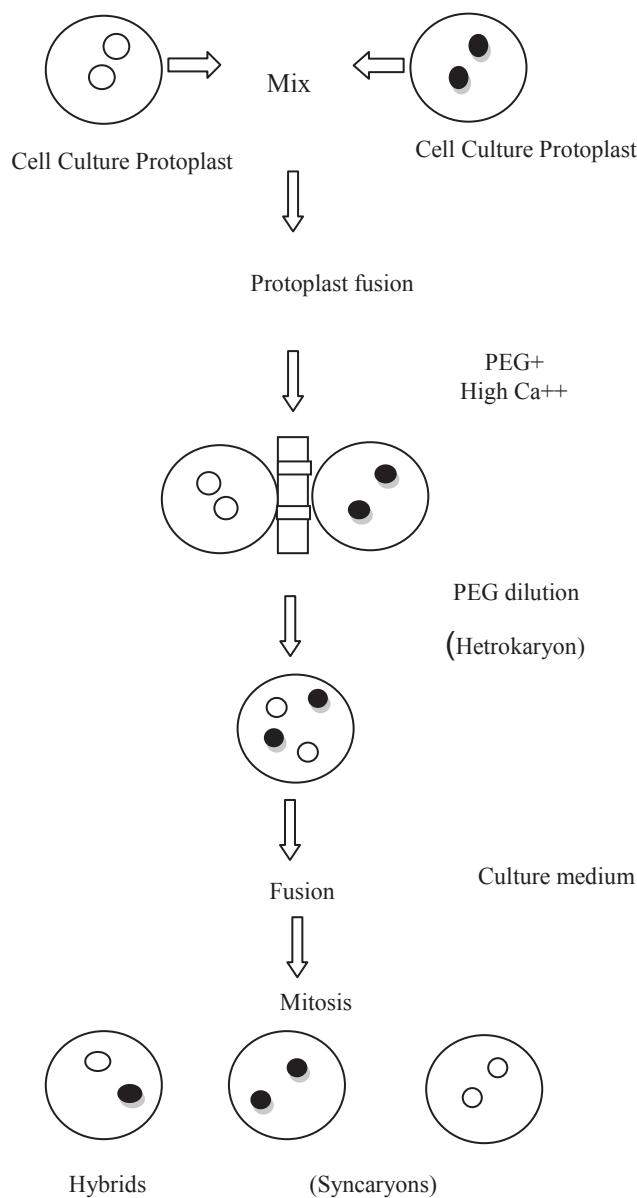
شکل ۳: ادغام پروتوپلاست
