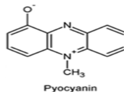
شکل ۱. ساختار پیوسیانین
