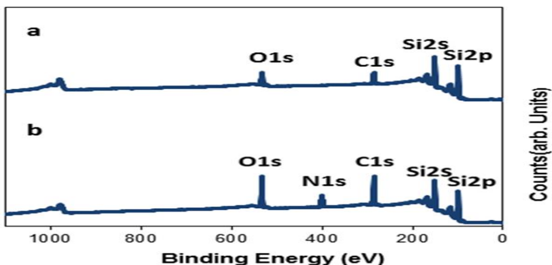
شکل ۳. طیف XPS بر روی سطح (a) ۸ نونادیان و (b) پپتید را نشان می دهد.
