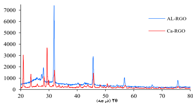
شکل ۲- طیف XRD نانوساختارهای Al/rGO و Ca/rGO
