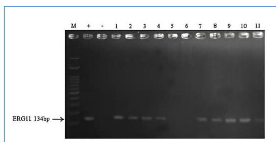
شکل ۱- باند DNA از قارچ کاندیدا/آلبیکس (M: نشانگر DNA
