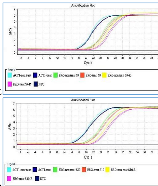
شکل ۵- A. منحنی ذوب ژن ERG11 ، B. میزان بیان ژن ERG11 در نمونه شماره ۱ نسبت به ژن ACT1 ، C. میزان بیان ژن ERG11 در نمونه شماره ۹ نسبت به ژن ACT1 ، D. میزان بیان ژن ERG11 در نمونه شماره ۱۰ نسبت به ژن ACT1
