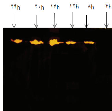
شکل ۳- بررسی نوع آنزیم تولید شده بر حسب زمان های مختلف کشت
