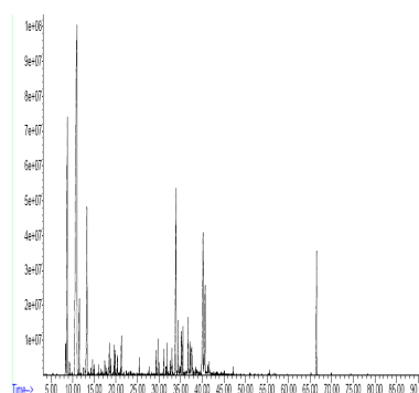
شکل ۸- طیف کروماتوگرام حاصل از اسانس Teucrium polium واقع
