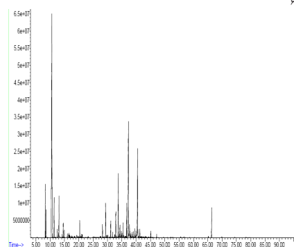
شکل ۷- طیف کروماتوگرام حاصل از اسانس Teucrium polium واقع
