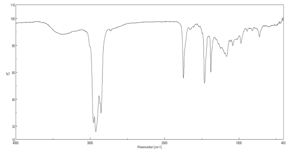
شکل ۳- گراف FTIR مربوط به روغن تک یاخته تولیدی توسط مخمر ژئوتریکوم BL
