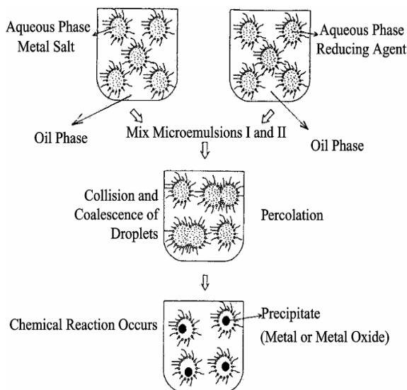
شکل ۴) شمایی از روش میکرومولسیون
