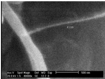
شكل ۷- تصاویر SEM الیاف باکتریال سلولز تشکیل شده در بزرگنمايى ۴۰۰۰۰ با قطر ۹۹ نانومتر (تصویر بالا) و ۴۱ نانومتر (تصویر پایین)
