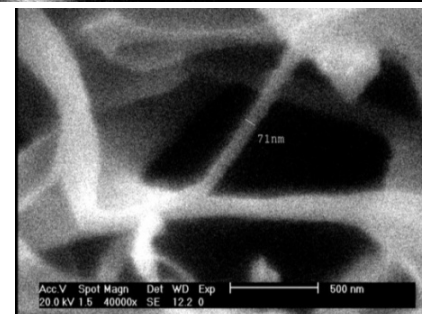
شكل ۶- تصاویر SEM گرفته شده در بزرگنمايى ۸۰۰۰۰ (بالا) تصویر و بزرگنمايى ۴۰۰۰۰ (پایین) که الیافی با قطر ۷۱ نانومتر را نشان می دهد.
