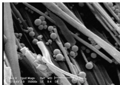
شکل-۲ تصویر SEM از نانوذره A۲ (بزرگنمایی ۱۵۰۰۰×)
