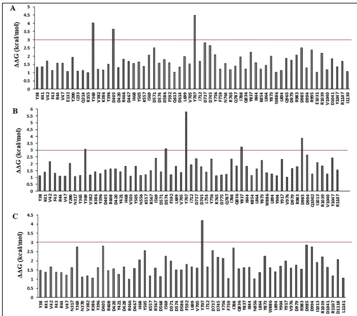
شکل ۲. اسیدهای آمینه هات اسپات در منطقه رابط بین مونومرها در SARS-CoV-2 (A) زیر واحد A، (B) زیر واحد B و (C) زیر واحد C. اسیدهای آمینه حاوی \Delta\Delta G \geq 3 به عنوان هات اسپات قرمز شناخته می‌شوند
