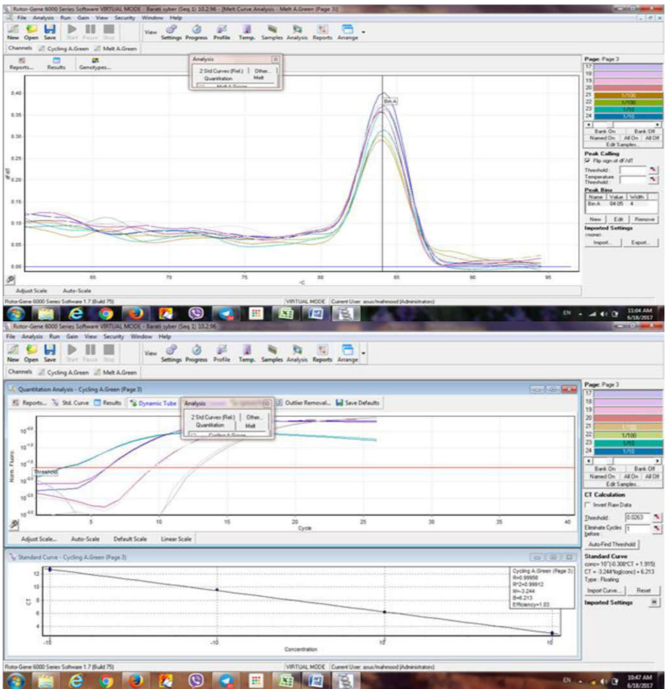
شکل ۳- روش Real-Time PCR با استفاده از رنگ SYBR Green در عامل بورخولدریا، نتیجه Real-Time PCR با دستگاه Corbett Rotorgen 6000 با استفاده از رنگ SYBR Green مربوط به واکنش پرایمر پیشرو و پیرو توالی بورخولدریا در غلظت و رقت‌های مختلف ۱۰۰ پیکوگرم، ۱۰ پیکونانوگرم، ۱ پیکوگرم و ۰/۱ پیکوگرم پلاسمید همراه نمودار standard curve و نمودار منحنی ذوب مربوطه نکته: هر واکنش به صورت دوگانه انجام شده است و هم‌چنین دارای نمونه کنترل منفی نیز است.
