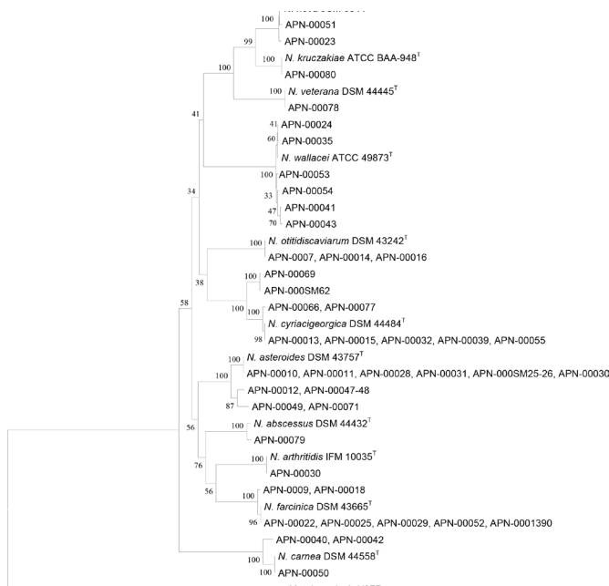
تصویر شماره ۲: درخت تکاملی و رابطه فیلوژنتیکی ایزوله های مورد بررسی در این مطالعه بر اساس MLSA توالی ژن های rRNA ۱۶S، gyrB ، secA
