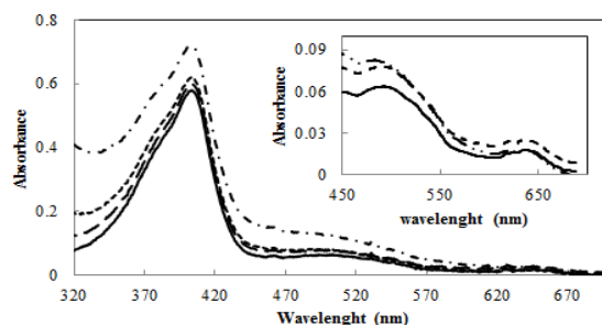
شکل ۴. طیف جذبی آنزیم پراکسیداز ترب کوهی در حضور غلظت های ۰ (خط پیوسته)، ۱۰۰ (خط چین)، ۳۰۰ (نقطه چین) و ۵۰۰ میکرومولار (خط-نقطه) کلرید روی. غلظت ۷۰۰ میکرومولار به دلیل احتمال وجود اگریگاسیون آورده نشده است.
