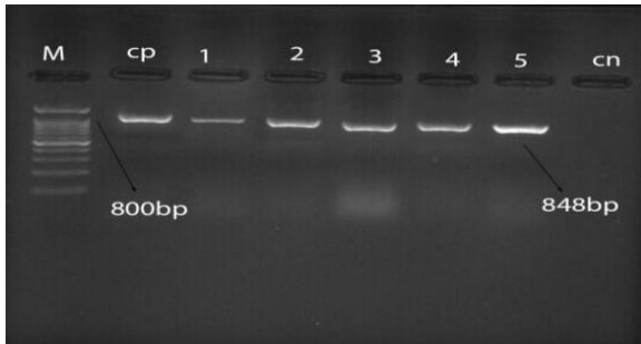
شکل ۳- الکتروفورز ژل آگارز ۱/۵٪ محصول PCR ژن TEM ستون M ۱۰۰bp DNA ladder، CP کنترل مثبت، CN کنترل منفی، ستون های ۱-۵ باند اختصاصی ۸۴۸ bp ژن TEM
