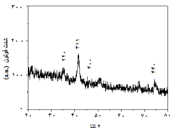
شکل ۱- منحنی پراش پرتو ایکس نانوذرات اکسید آهن سنتز شده به روش سبز، اندازه نانوذرات را ۱۵ نانومتر نشان داد
