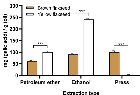
شکل ۲- مقدار ترکیب‌های فنولی روغن استخراج شده با روش حلال و پرس سرد. آزمون سه بار تکرار و نتایج به صورت میانگین \pm خطای استاندارد گزارش شده است ( p < 0.001 : ***).
