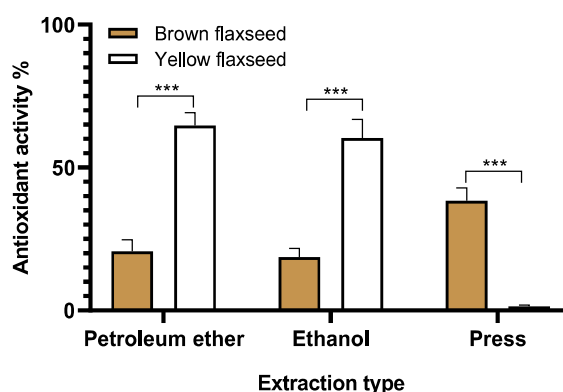
شکل ۳- فعالیت آنتی اکسیدانی روغن استخراج شده از کتان زرد و قهوه‌ای با روش حلال و پرس. آزمون سه بار تکرار و نتایج به صورت میانگین \pm خطای استاندارد گزارش شده است (***: p < 0.001 ).
