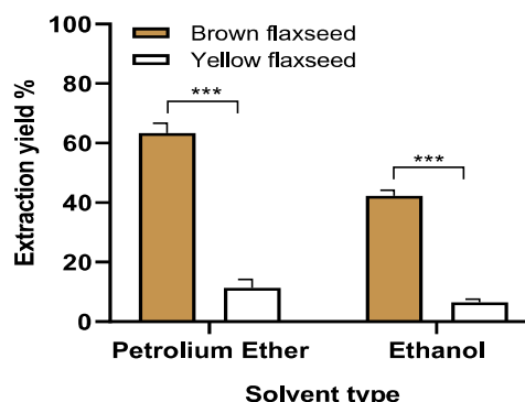
شکل ۱- بازده روغن استخراج شده از دو نوع کتان زرد و قهوه‌ای با دو نوع حلال. همان‌طور که دیده می‌شود میزان روغن استخراج شده از دانه کتان قهوه‌ای با استفاده از هر دو حلال به‌طور معنی‌داری بیش‌تر از میزان روغن استخراج شده از دانه کتان زرد است. آزمون سه بار تکرار و نتایج به صورت میانگین \pm خطای استاندارد گزارش شده است.
