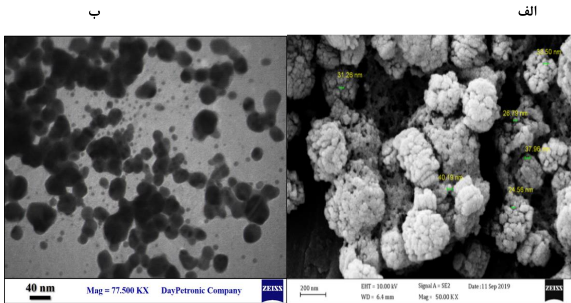
شکل ۵: نتایج میکروسکوپ الکترونی (الف) نگاره (SEM): همانطور که مشاهده می‌شود نانوذرات سنتز شده دارای ساختاری کروی و دارای میانگین اندازه ۳۳/۵ نانومتر می‌باشد. (ب) نگاره (TEM)
