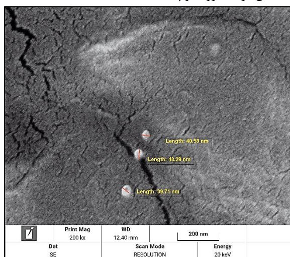
تصویر ۱- تصویر FE-SEM از نانوسامانه نیوزومی پگیله قبل از بارگذاری دارو
