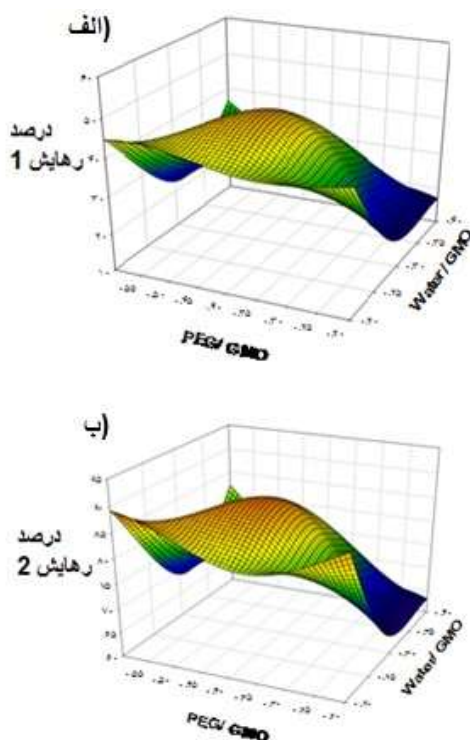
شکل ۴- نمودار سه بعدی (الف) درصد رهایش ۱ (ب) درصد رهایش ۲ با نسبت‌های وزنی PEG/GMO و Water/GMO در مقدار ثابت الانزایین
