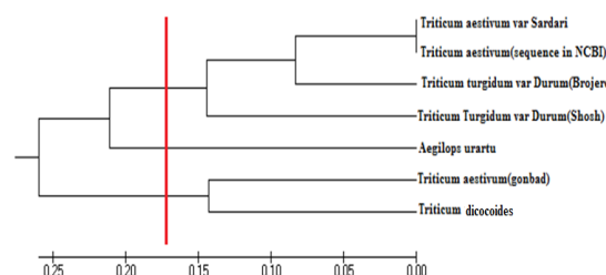
شکل ۴- دندوگرام حاصل از تأثیر آنزیم های برشی بر ژن Wdhn۱۳ گونه های گندم دارای ژن (Wdhn۱۳) مورد بررسی از روش NJ توسط نرم افزار MEGA۵.
