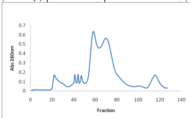
شکل ۱- منحنی جذب در ۲۸۰ نانومتر به فراکشن های مختلف
