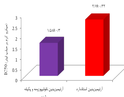
شکل ۳: مقادیر IC_{50} (μg/ml) برای فرمولاسیون های داروی نانولیپوزوم ی
