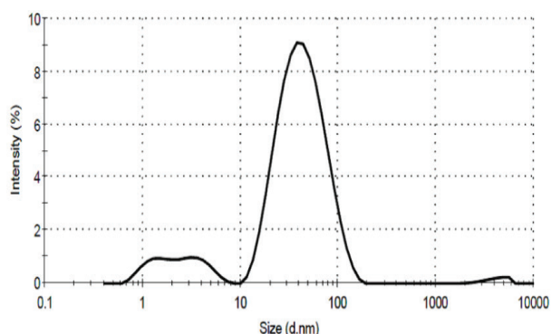
شکل ۲. نتیجه ی DLS نانوذرات طلا
