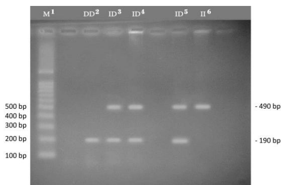
شکل ۱- تصویر ژل تهیه شده از الکتروفورز PCR
