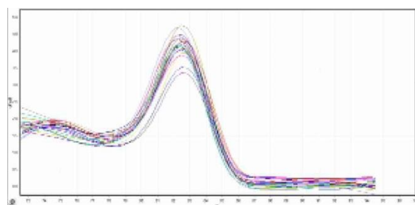
نمودار ۲. منحنی ذوب VEGFA
