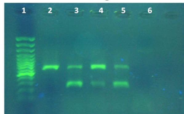
شکل ۴. الکتروفورز نتایج PCR با تعداد مشخص DNA ویروس هپاتیت B و حاوی اینترنال کنترل:
