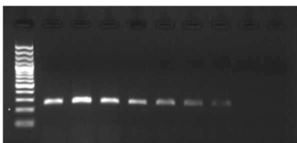
شکل ۱. تست حساسیت PCR با استفاده از نمونه های حاوی تعداد
