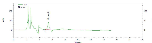
شکل ۱. کروماتوگرام طیف نمونه استاندارد هایپرسین
